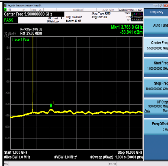
NTNV-N7-PC3-15-25-L-DFT-QPSK-Edge_1RB_L eft-Ant1-PASS
