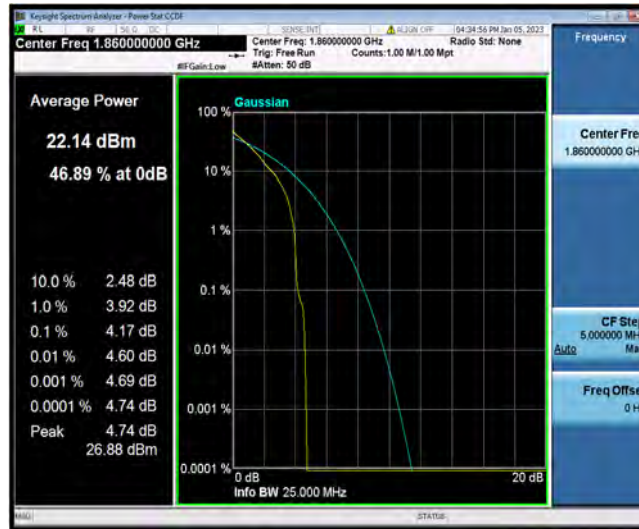
N25-20MHz-QPSK-372000-100RB#0
