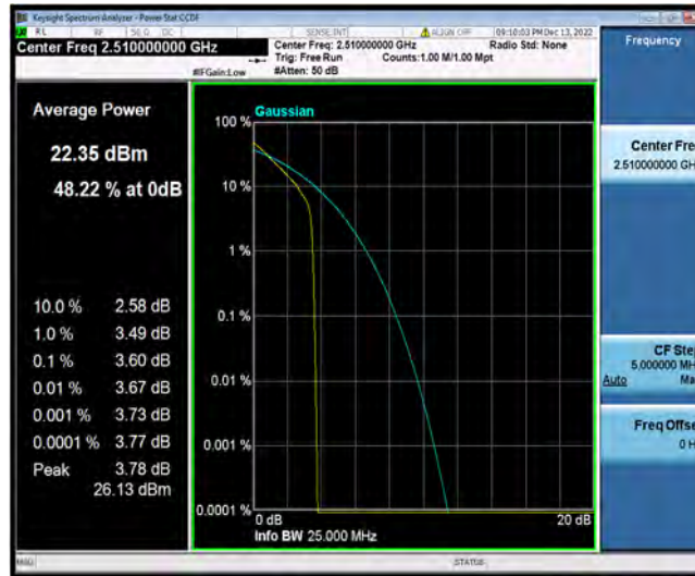
N7-20MHz-QPSK-502000-100RB#0
