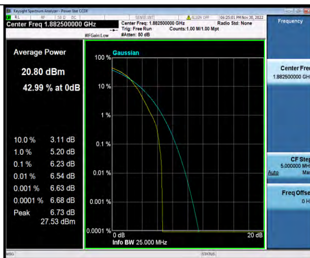
Band25-20MHz-64QAM-26365-100RB#0
