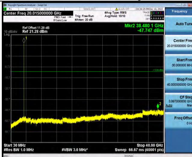
Band42-5MHz-QPSK-42590-1RB#0-Range1:30~40000MHz
