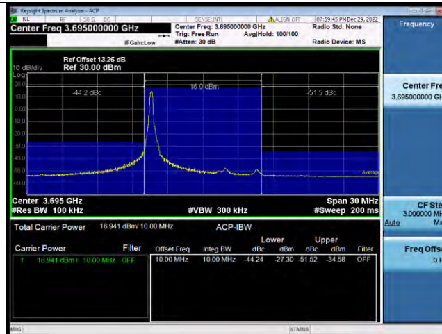
Band48-10MHz-QPSK-56690-50RB#0
