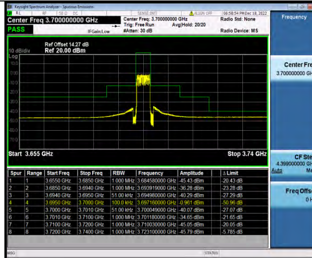
Band48-10MHz-QPSK-55290-1RB#0
