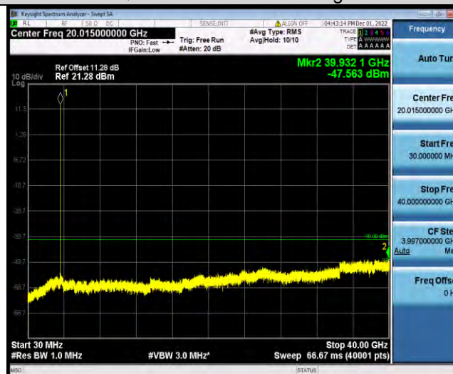
Band48-10MHz-QPSK-56690-1RB#0-Range1:30~40000MHz
