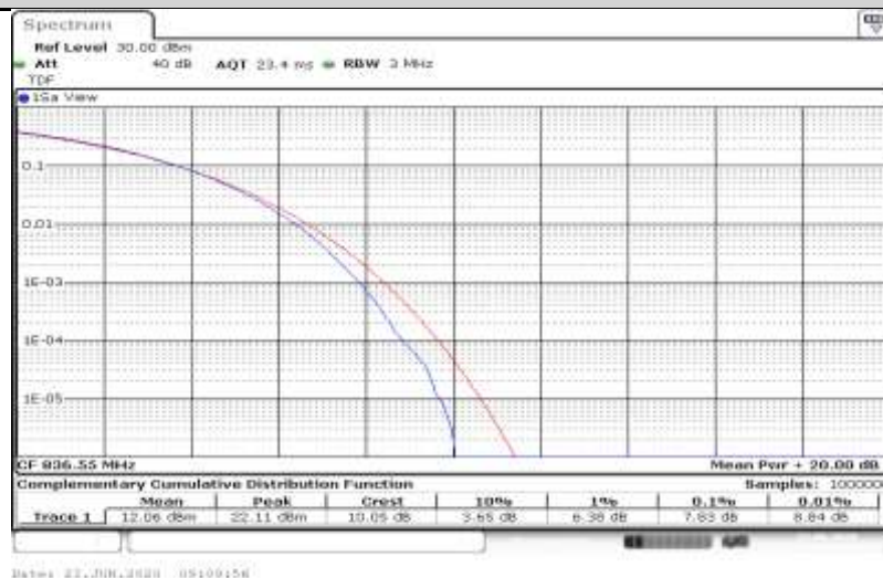
5-5-10MHz-10MHz-QPSK-20501-20600-50RB#0-50RB#0
