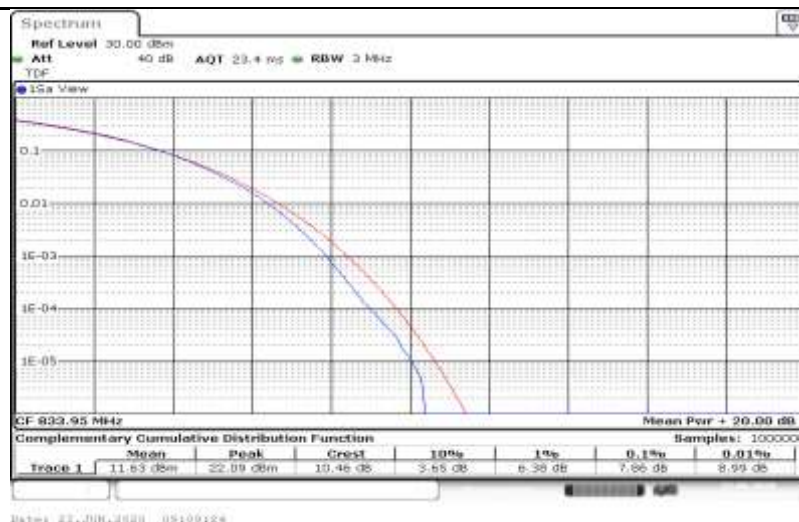
5-5-10MHz-10MHz-QPSK-20476-20575-50RB#0-50RB#0
