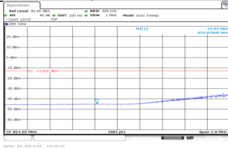
5-5-MHz-10MHz-QPSK-20428-20500-25RB#0-50RB#0
