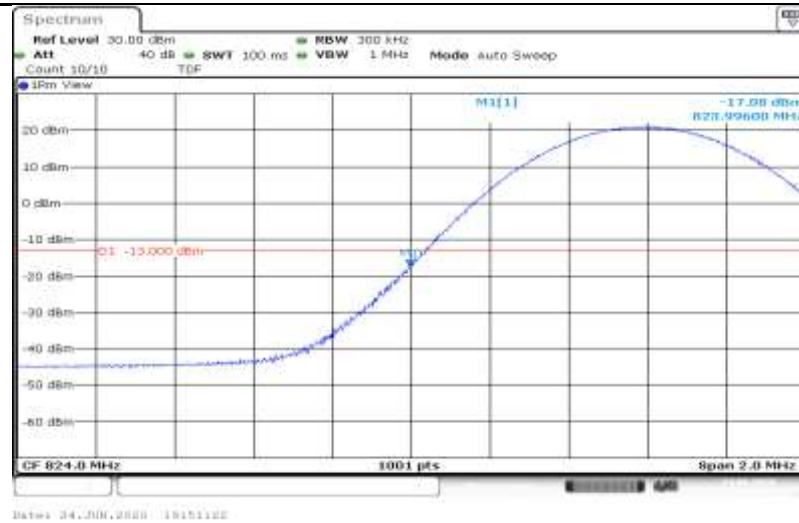
5-10MHz-10MHz-16QA M-20450-20549-50RB#0-50RB#0
