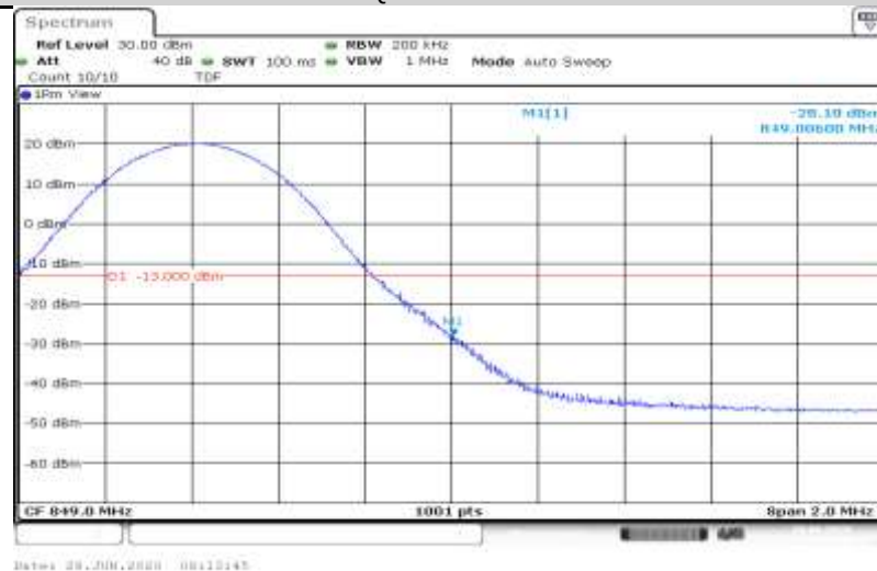
5-10MHz-10MHz-16QA M-20501-20600-50RB#0-50RB#0
