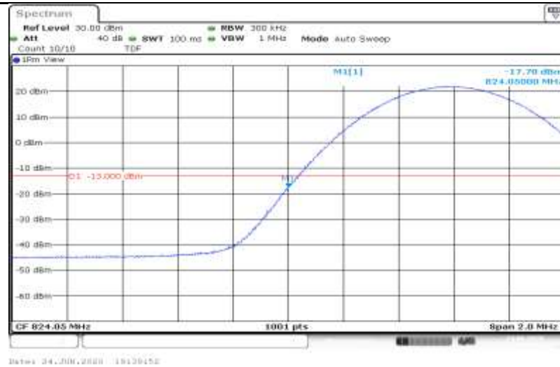
5-5-MHz-10MHz-QPSK-20428-20500-1RB#24-0RB#0
