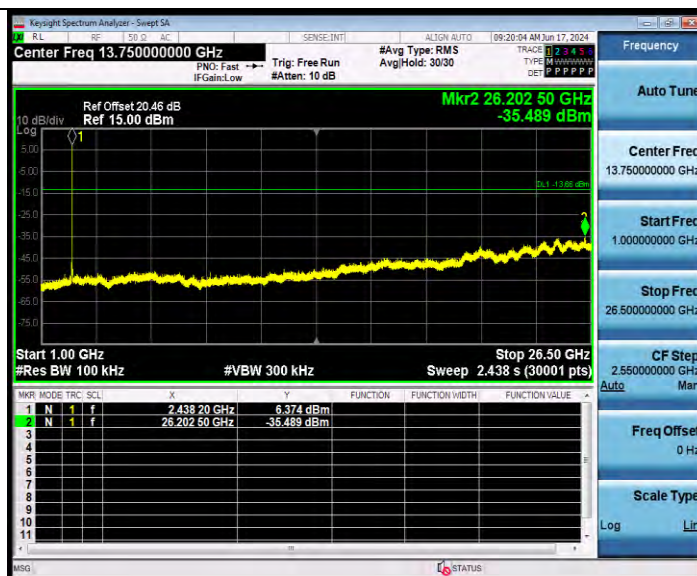
11B-CDD_Ant2_2437_0~Reference
