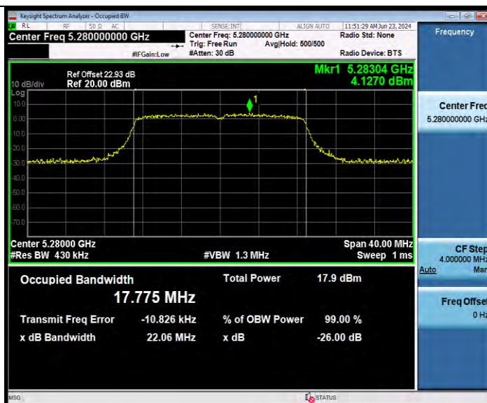
11N20MIMO Ant2 5280
