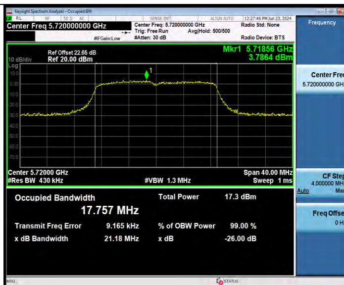
11N20MIMO Ant2 5720
