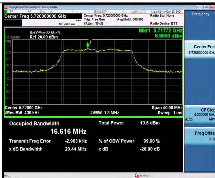
11A-CDD Ant2 5720
