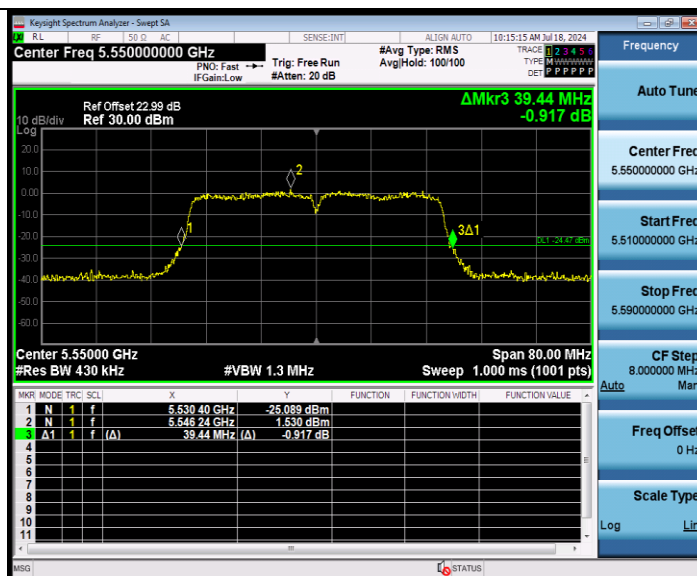
11N40MIMO Ant2 5550
