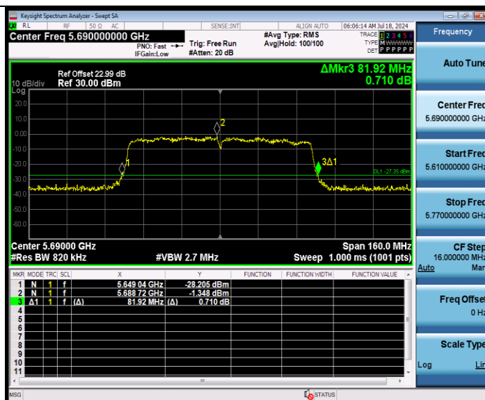
11AC80MIMO_Ant2_5690
