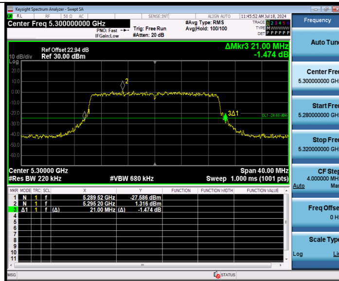
11AX20MIMO_Ant2_5300
