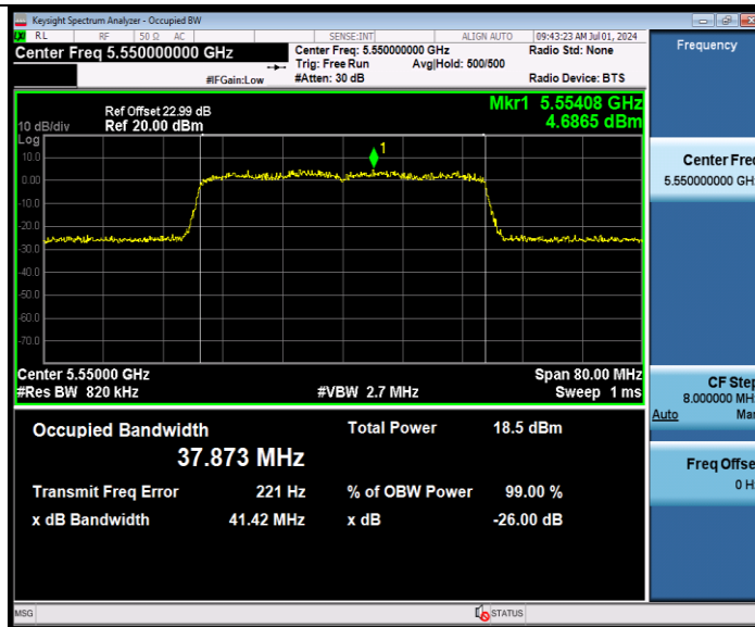
11AX40MIMO_Ant2_5550
