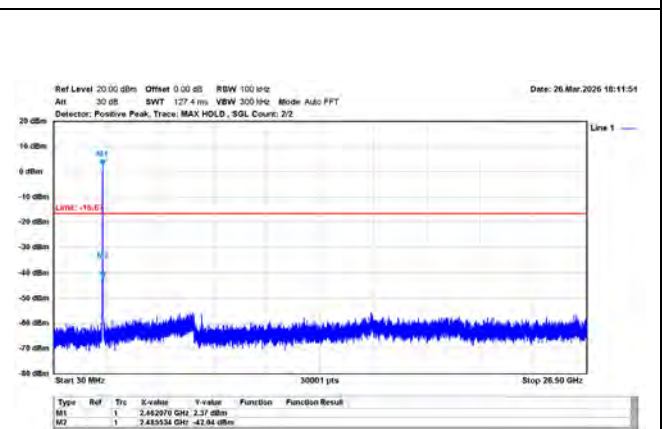
802.11n/20MHz/MCS0/2462MHz/Ch11/Ant.1
