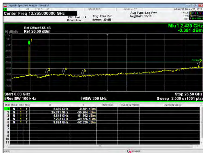
Tx. Spurious NVHT n40 2452MHz Ant1 Ref
