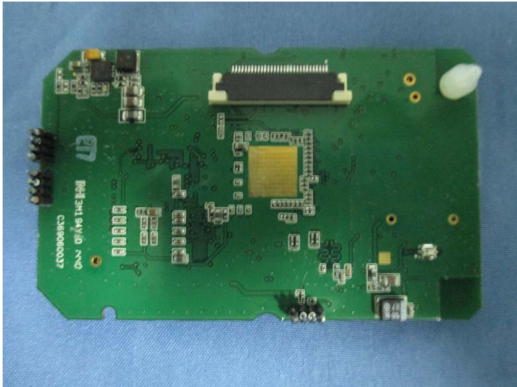
(16) EUT Photo (5GHz)
