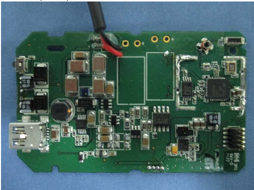
(10) EUT Photo (2.4GHz)
