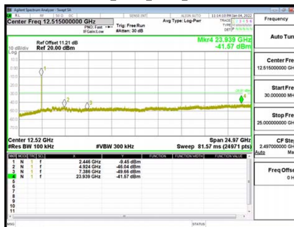
802.11n_40MHz_Chain1_2462MHz
