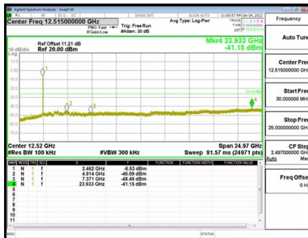
802.11n_40MHz_Chain0_2462MHz
