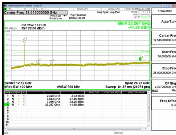
802.11n_40MHz_Chain1_2422MHz
