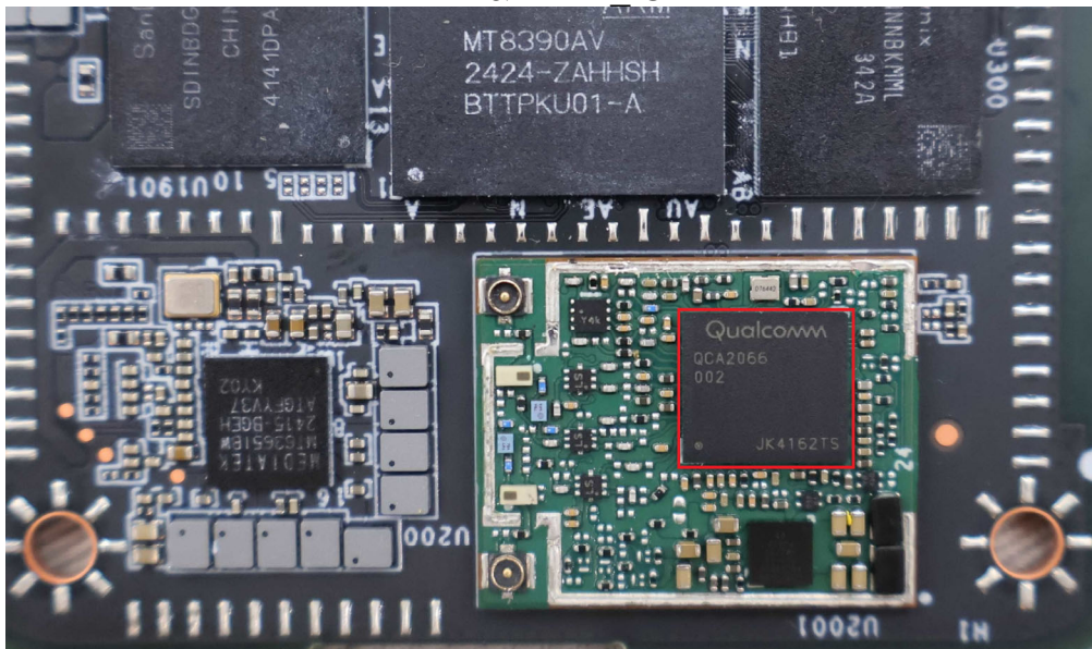
BT&WLAN IC
