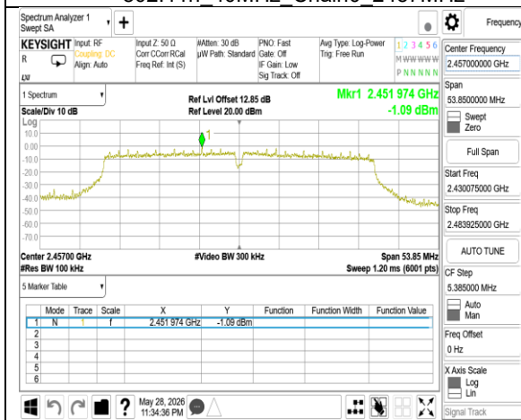
802.11n 40MHz Chain1 2457MHz
