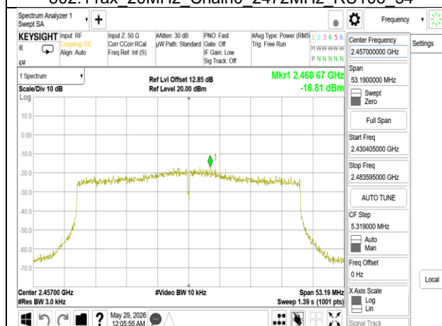
802.11ax 40MHz Chain0 2457MHz
