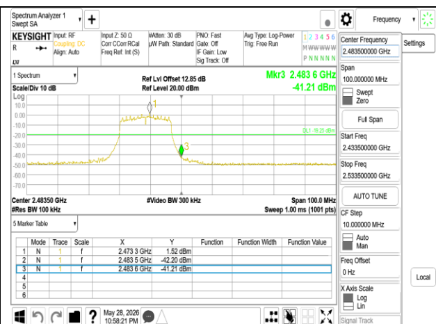
802.11g_20MHz_Chain1_2472MHz
