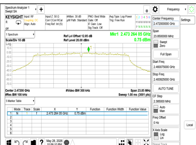
802.11g_20MHz_Chain1_2472MHz
