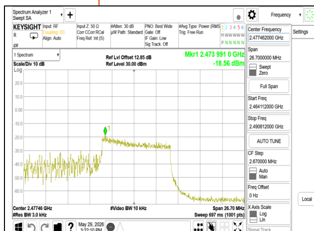
802.11ax 20MHz Chain0 2472MHz RU106 54
