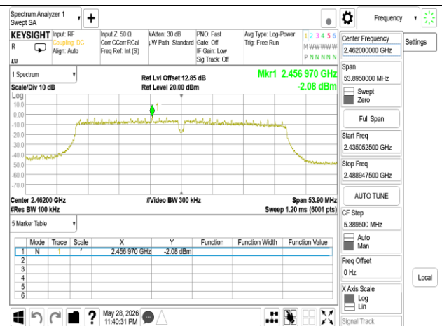
802.11n 40MHz Chain0 2462MHz
