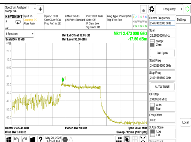
802.11ax 20MHz Chain1 2472MHz RU106 54
