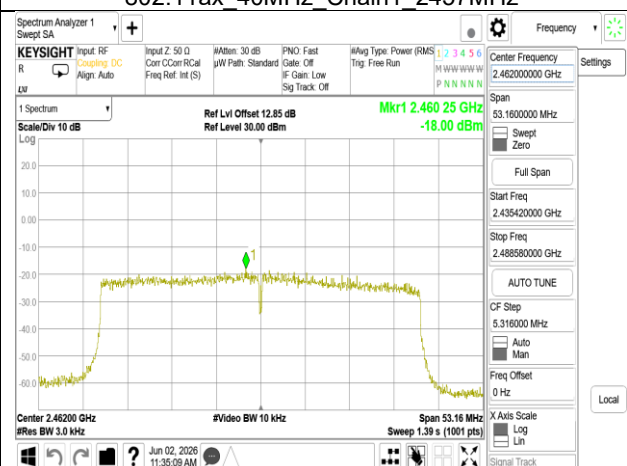
802.11ax 40MHz Chain1 2462MHz
