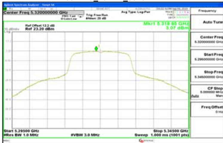
802.11a_20MHz_5320MHz
