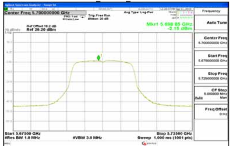
802.11a_20MHz_5700MHz
