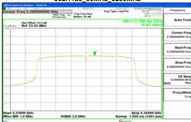
802.11ac_80MHz_5290MHz
