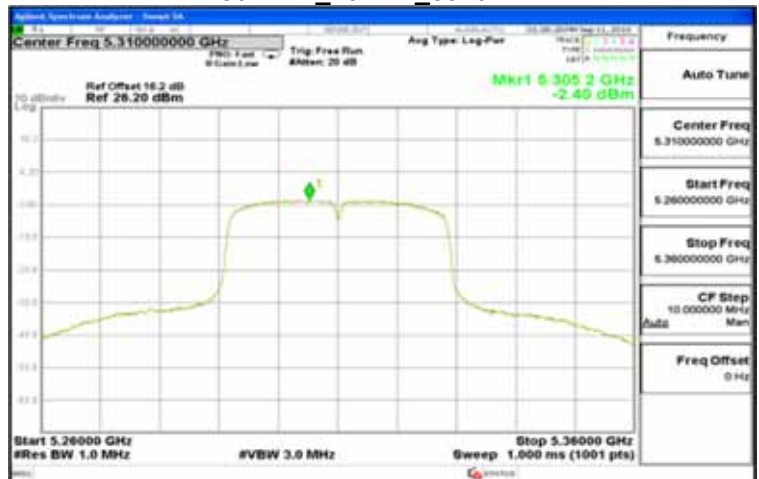
802.11n_40MHz_5310MHz
