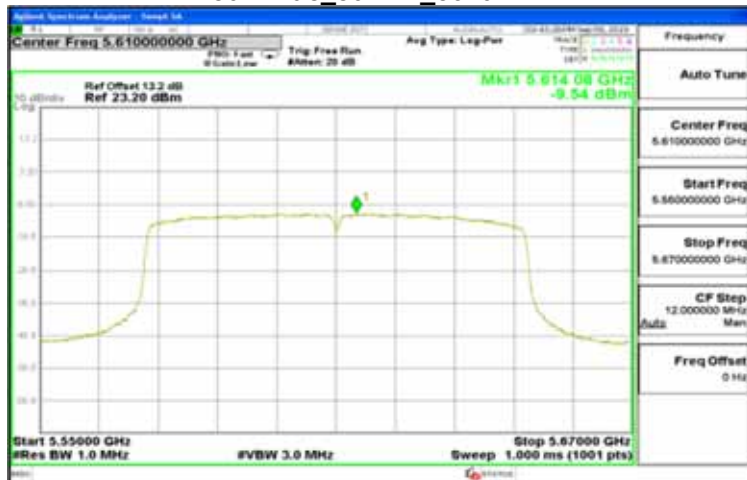
802.11ac_80MHz_5610MHz
