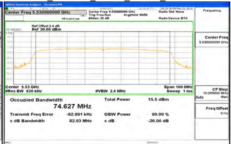
FCC 802.11ac 80MHz_Chain1_5530MHz
