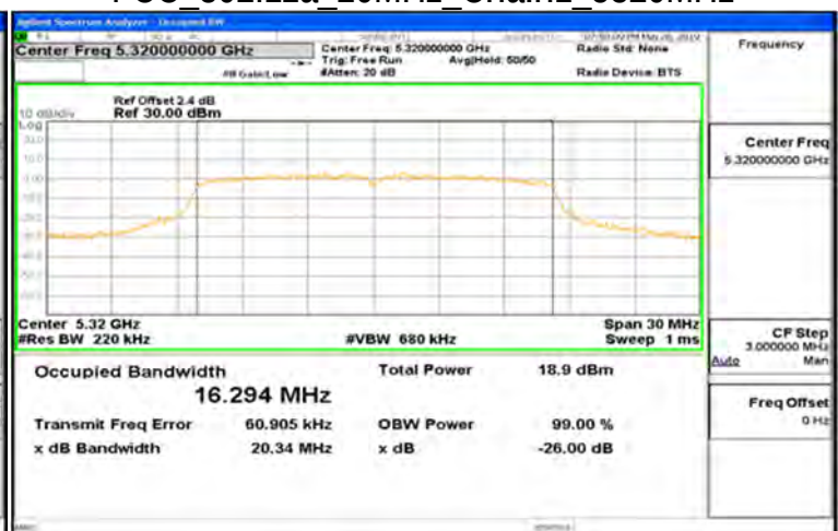
FCC 802.11a 20MHz_Chain1_5320MHz
