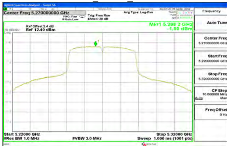
802.11n 40MHz 5270MHz
