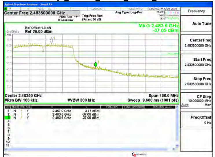
Band Edge 802.11n 40MHz Chain1 2452MHz
