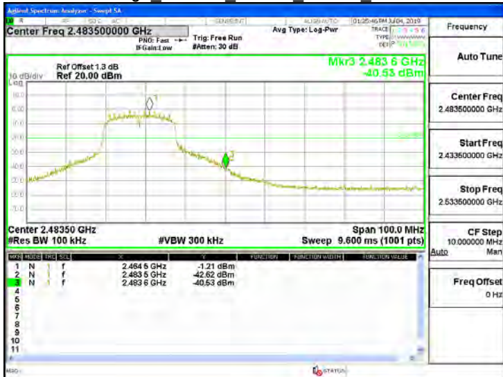
Band Edge 802.11n 20MHz Chain1 2462MHz
