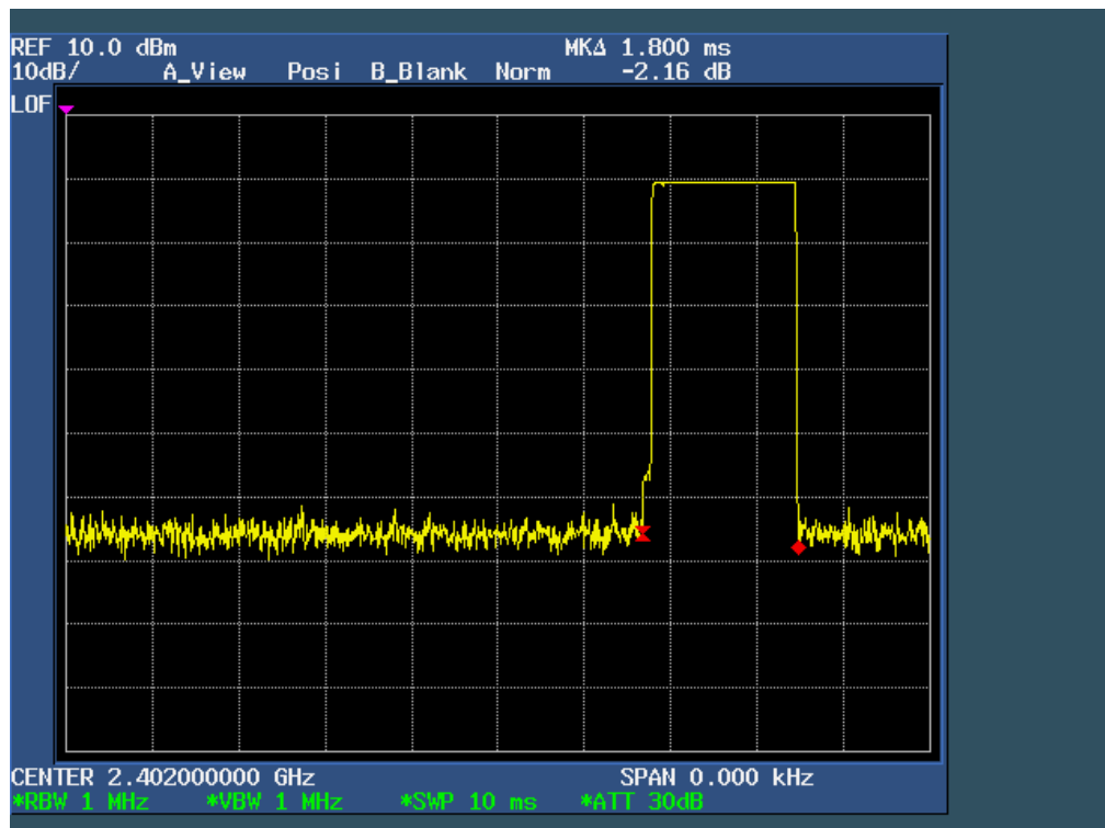
CH00-DH3
