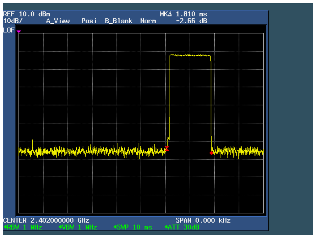
CH00-DH3
