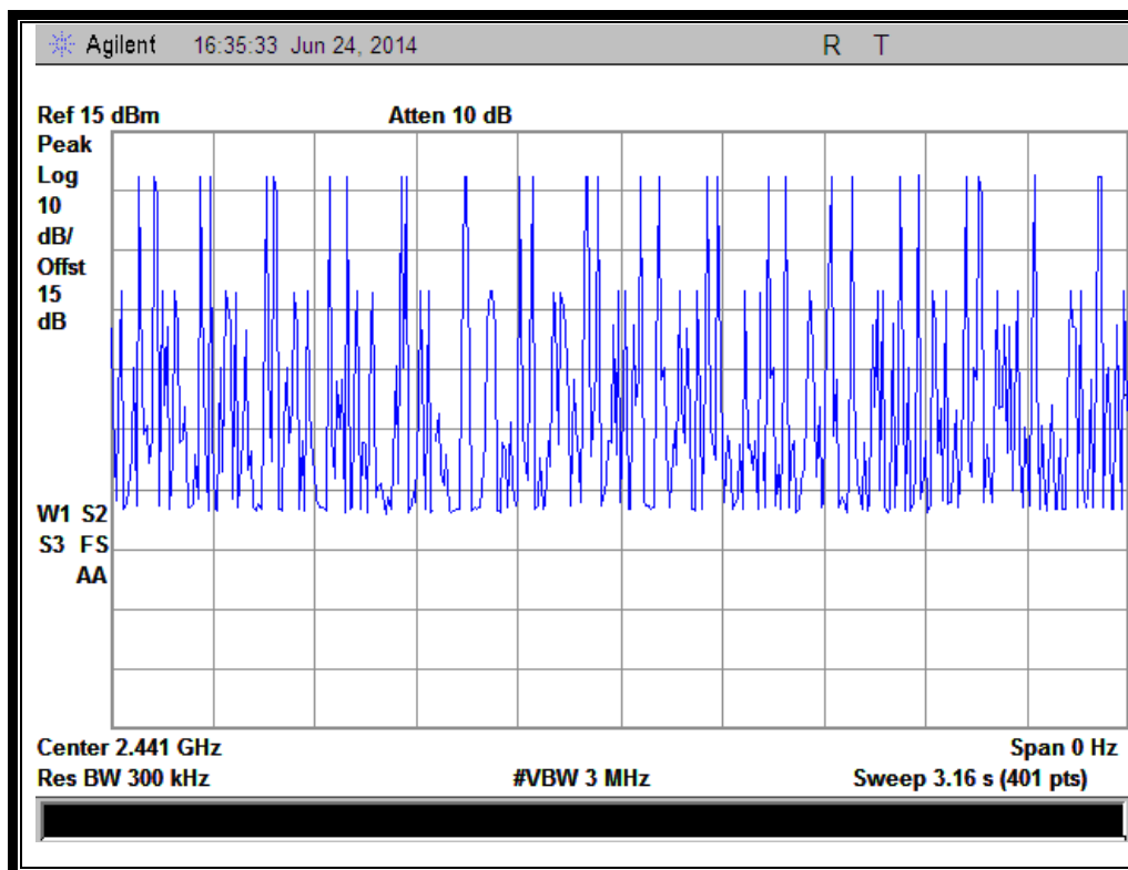
(Plot A: DH1 @ 8-DPSK)
