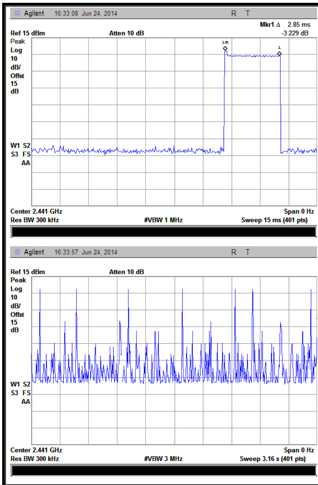
(Plot C: DH5 @ \pi/4 -DQPSK)
