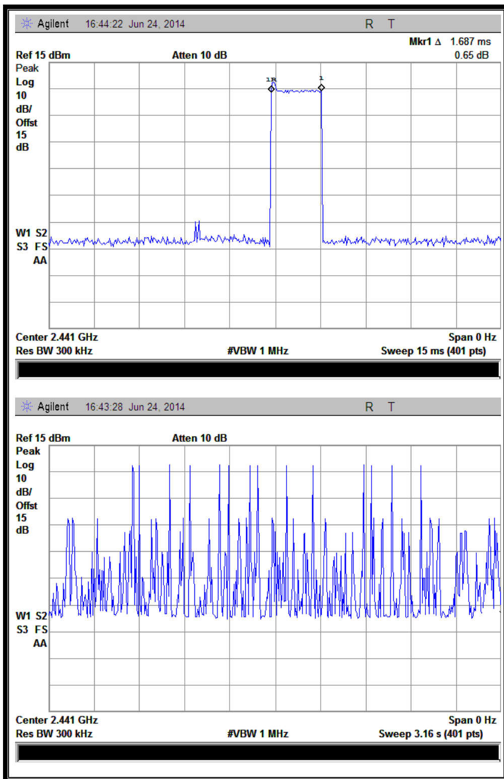
(Plot B: DH3 @ \pi/4 -DQPSK)
