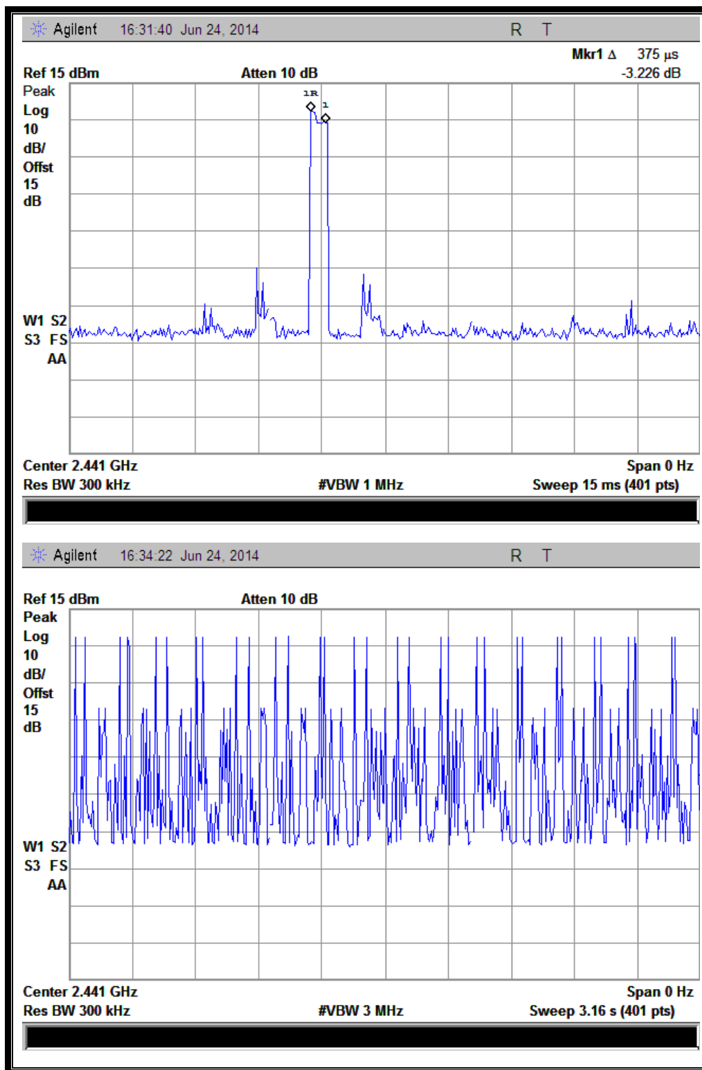
(Plot A: DH1 @ \pi/4 -DQPSK)
