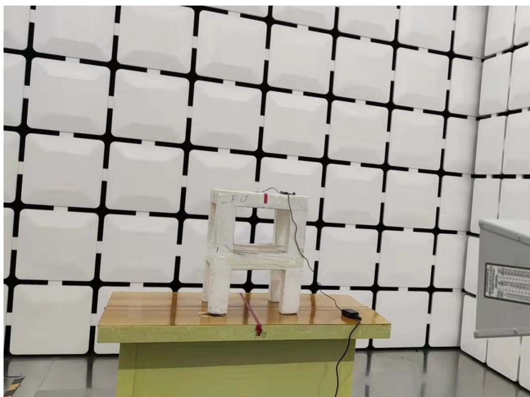
1GHz ~ 18GHz
