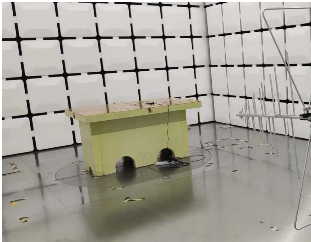
30MHz ~ 1GHz
