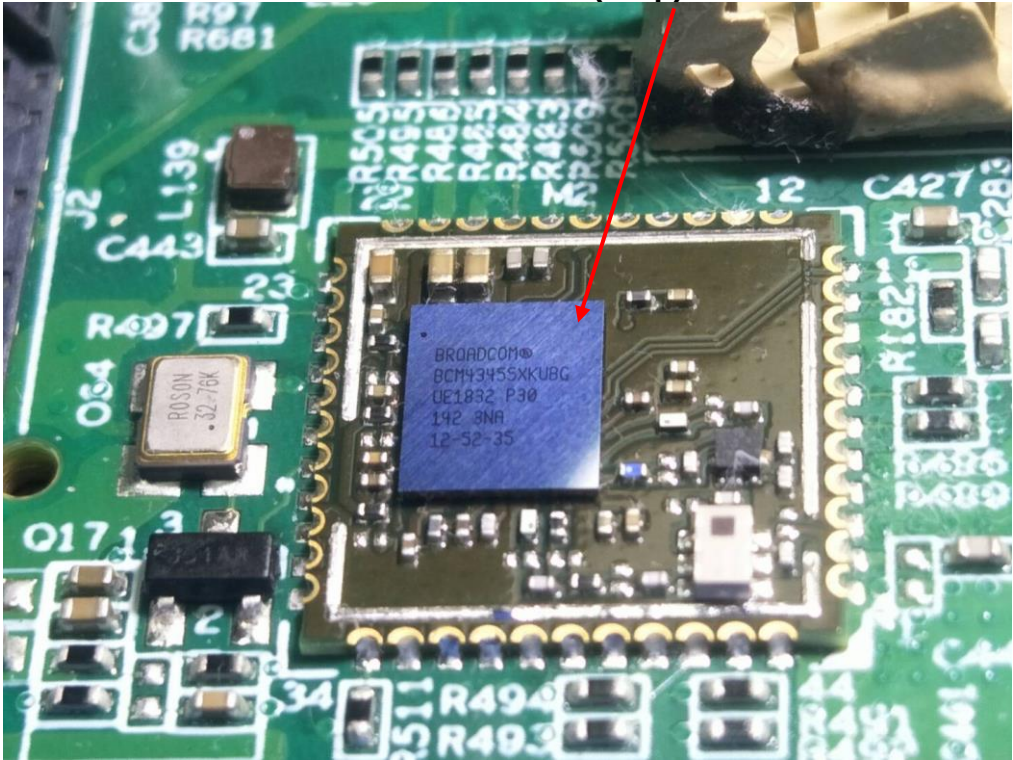
Wi-Fi/BT Module (Chip)
