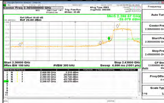
11N20MIMO_Ant1_Low_2412
