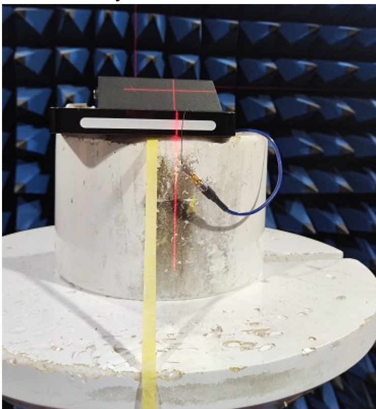
The production test position/天线测试放置位置
