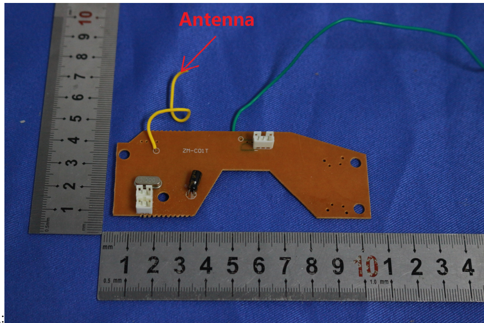
EUT Antenna:
