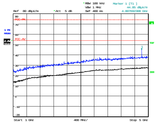
1GHz – 5GHz
