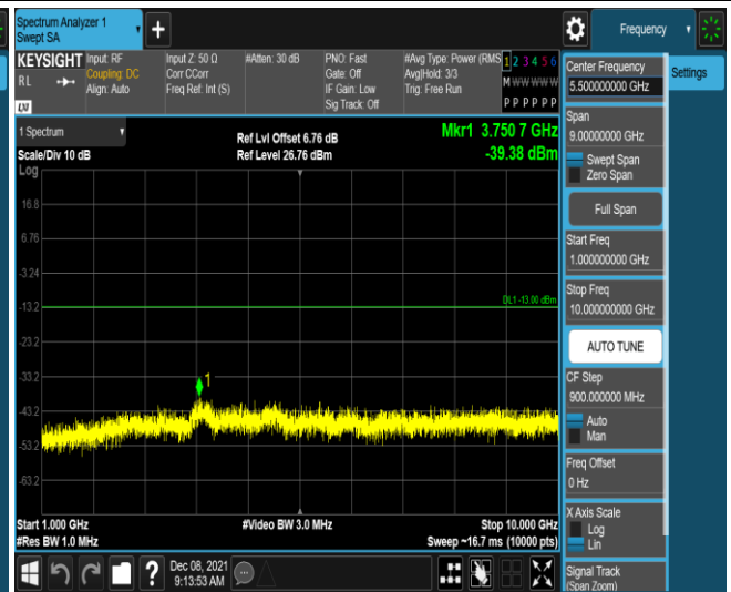
Band26-10MHz-QPSK-26740-1RB#0-Range2:1000~ 10000MHz
