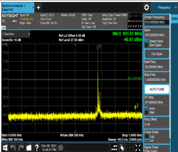
Band71-20MHz-QPSK-133372-1RB#0-Range1:30~1000MHz
