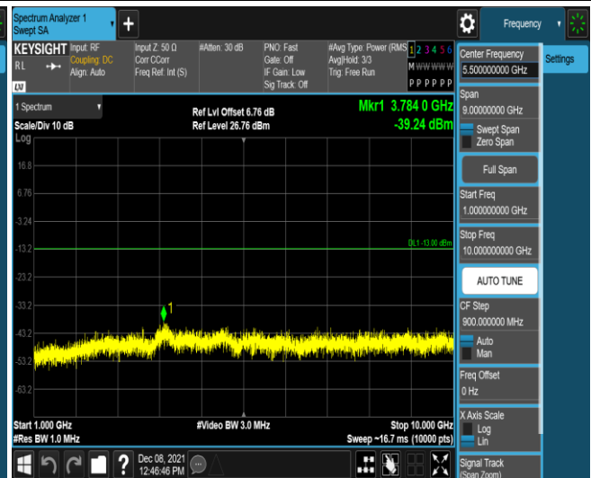
Band71-20MHz-QPSK-133372-1RB#0-Range2:1000~10000MHz
