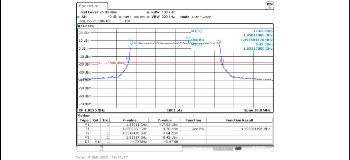
Band25-5MHz-QPSK-26365-25RB#0
