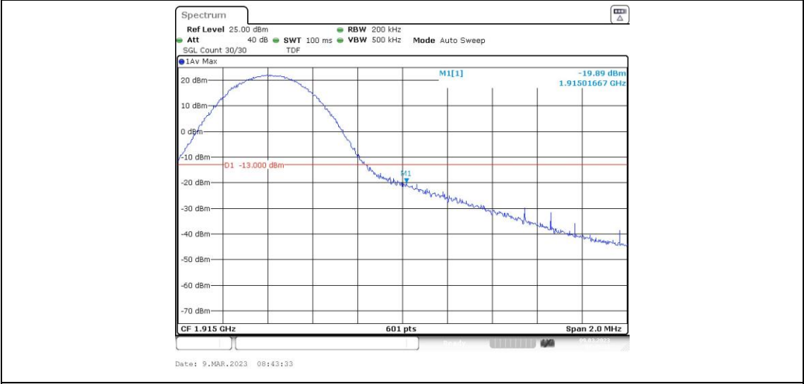
Band25-10MHz-QPSK-26640-50RB#0
