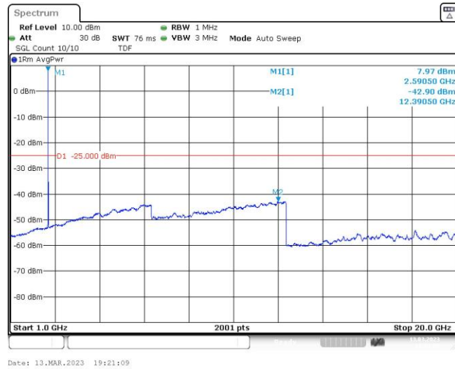
Band41-10MHz-QPSK-40640-1RB#0-Range5:20000~27000MHz
