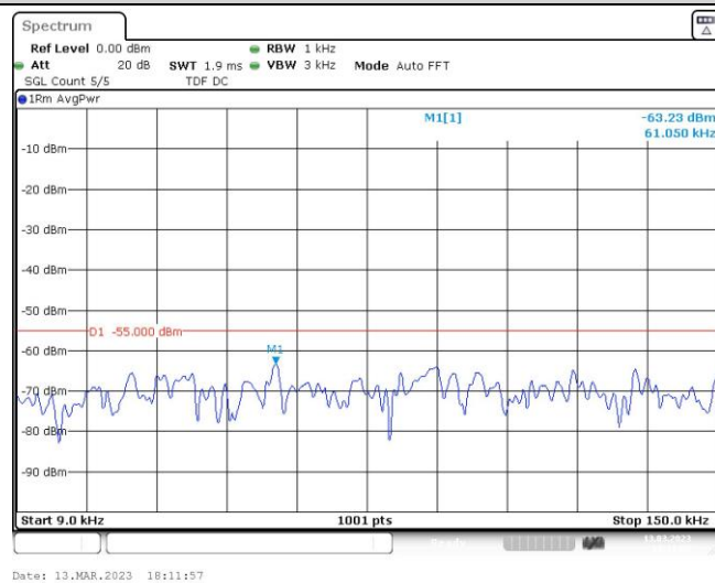
Band41-5MHz-QPSK-41215-1RB#0-Range2:0.15~30MHz
