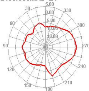
2450.000MHz E1
