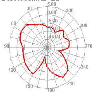
2450.000MHz E2
