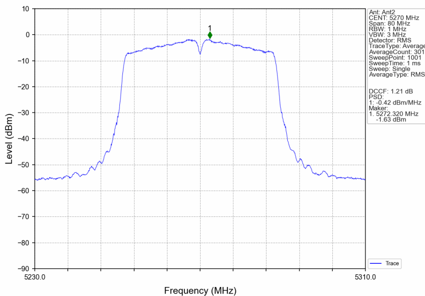
802.11n(HT40)_LCH_5270MHz_Ant2_NTNV
