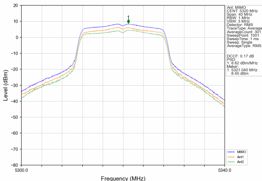
802.11a_HCH_5320MHz_MIMO_NTNV
