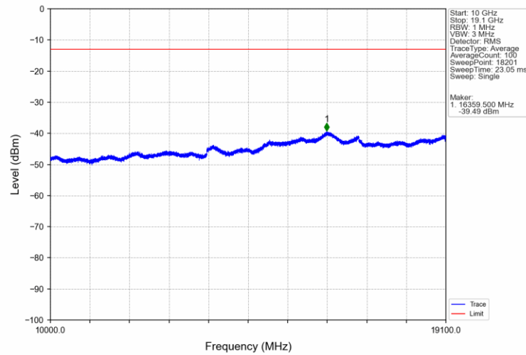
Band2_10MHz_QPSK_HCH_1905MHz_RB_1_49_NTNV
