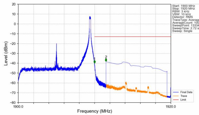
Band2_10MHz_QPSK_HCH_1905MHz_RB_1_49_NTNV
