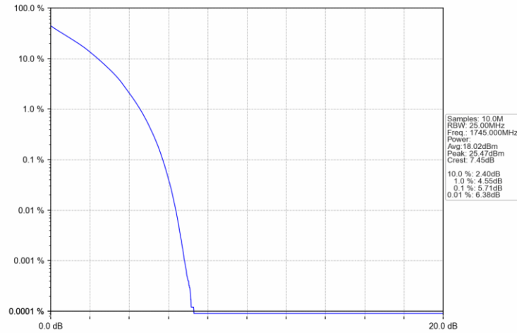
Band4 20MHz QPSK HCH 1745MHz RB 100 0 NTV
