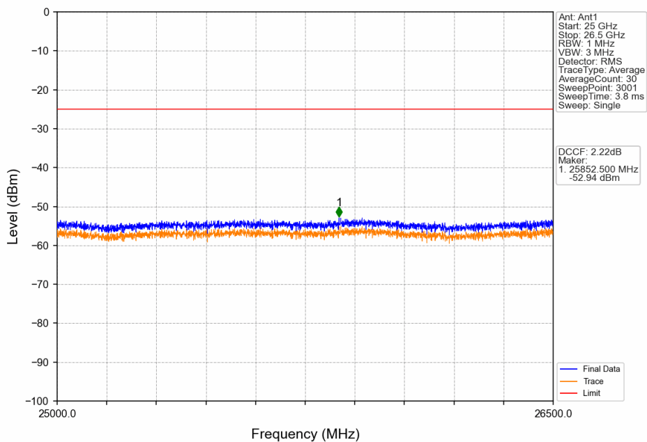
Band41_10MHz_16QAM_LCH_2560MHz_RB_50_0_NTNV
