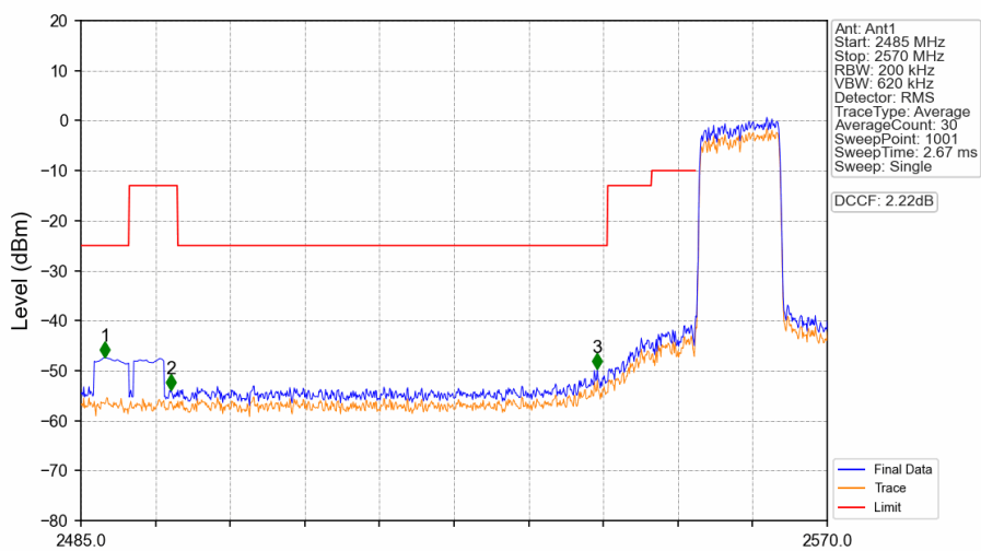
Band41_10MHz_16QAM_LCH_2560MHz_RB_50_0_NTNV
