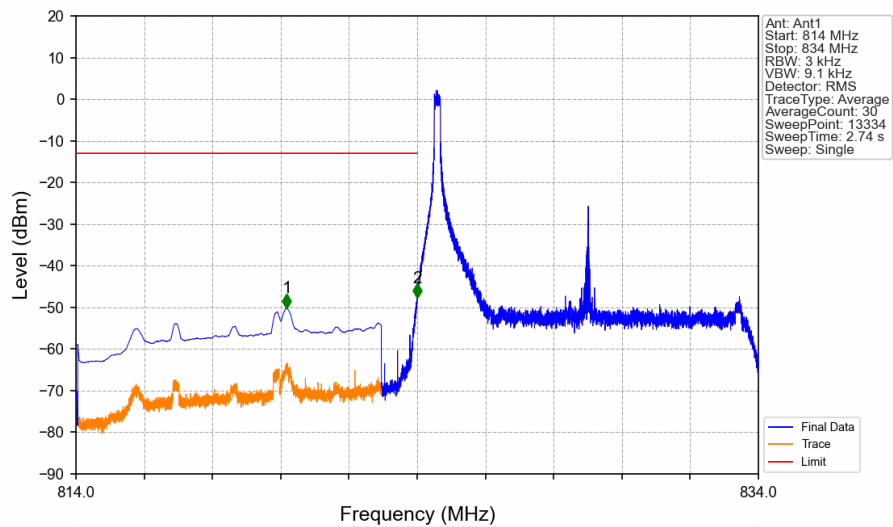
Band5_10MHz_QPSK_LCH_829MHz_RB_1_0_NTNV
