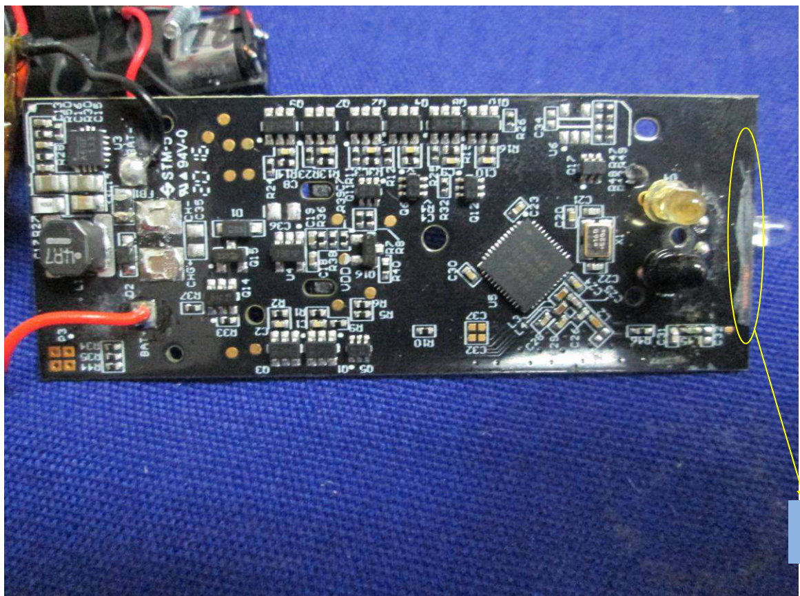
2.4G Antenna
