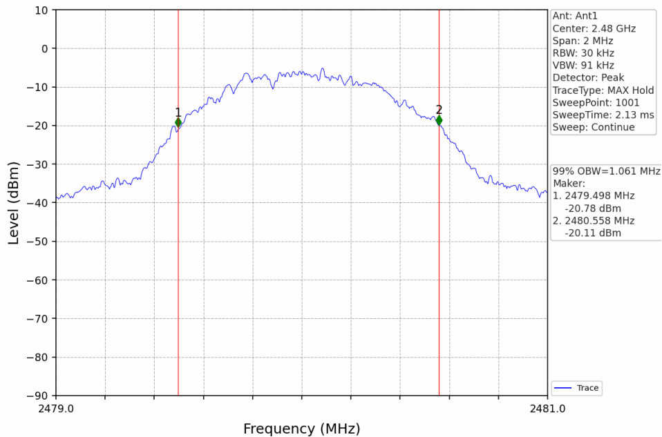
1M_HCH_2480MHz_DataRate=_Ant1_NTNV
