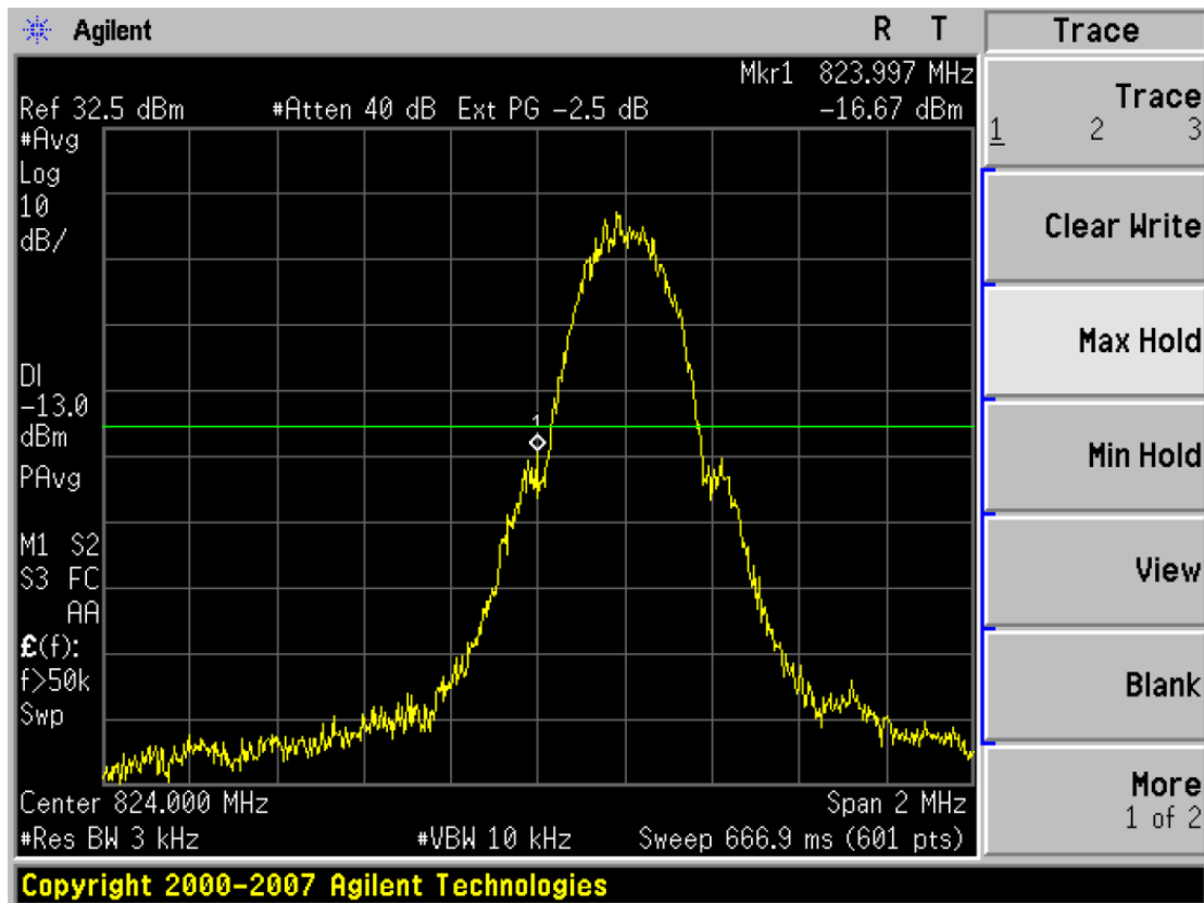
(Plot 4.4.1 A: Channel 128: 824.20MHz @ GSM850)
