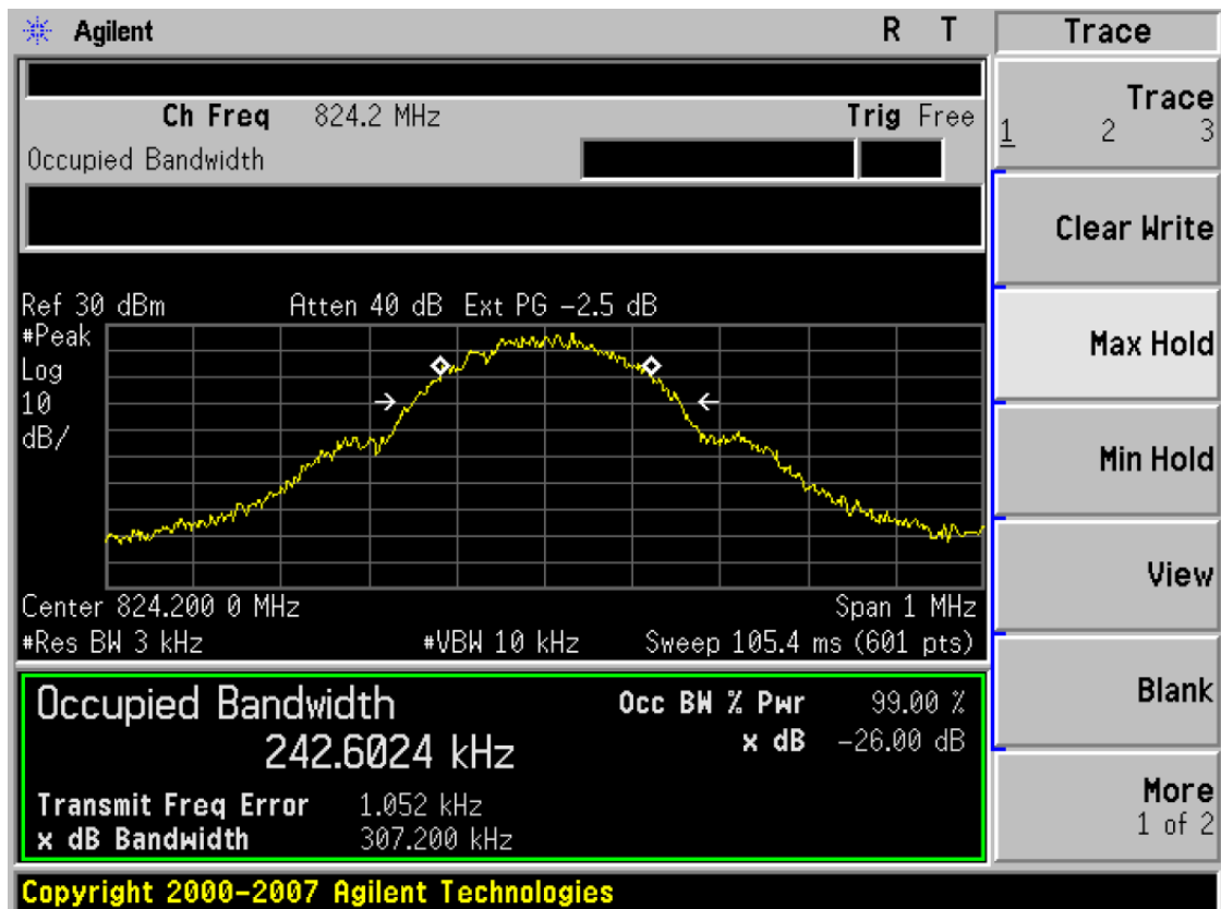
(Plot 4.3.1 A: Channel 128: 824.20MHz @ GSM850)
