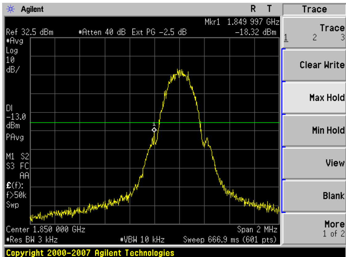
(Plot 4.4.3 A: Channel 512: 1850.20MHz @ PCS1900)
