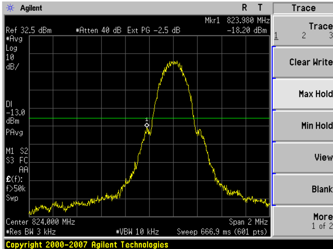
(Plot 4.4.2 A: Channel 128: 824.20MHz @ GPRS850)
