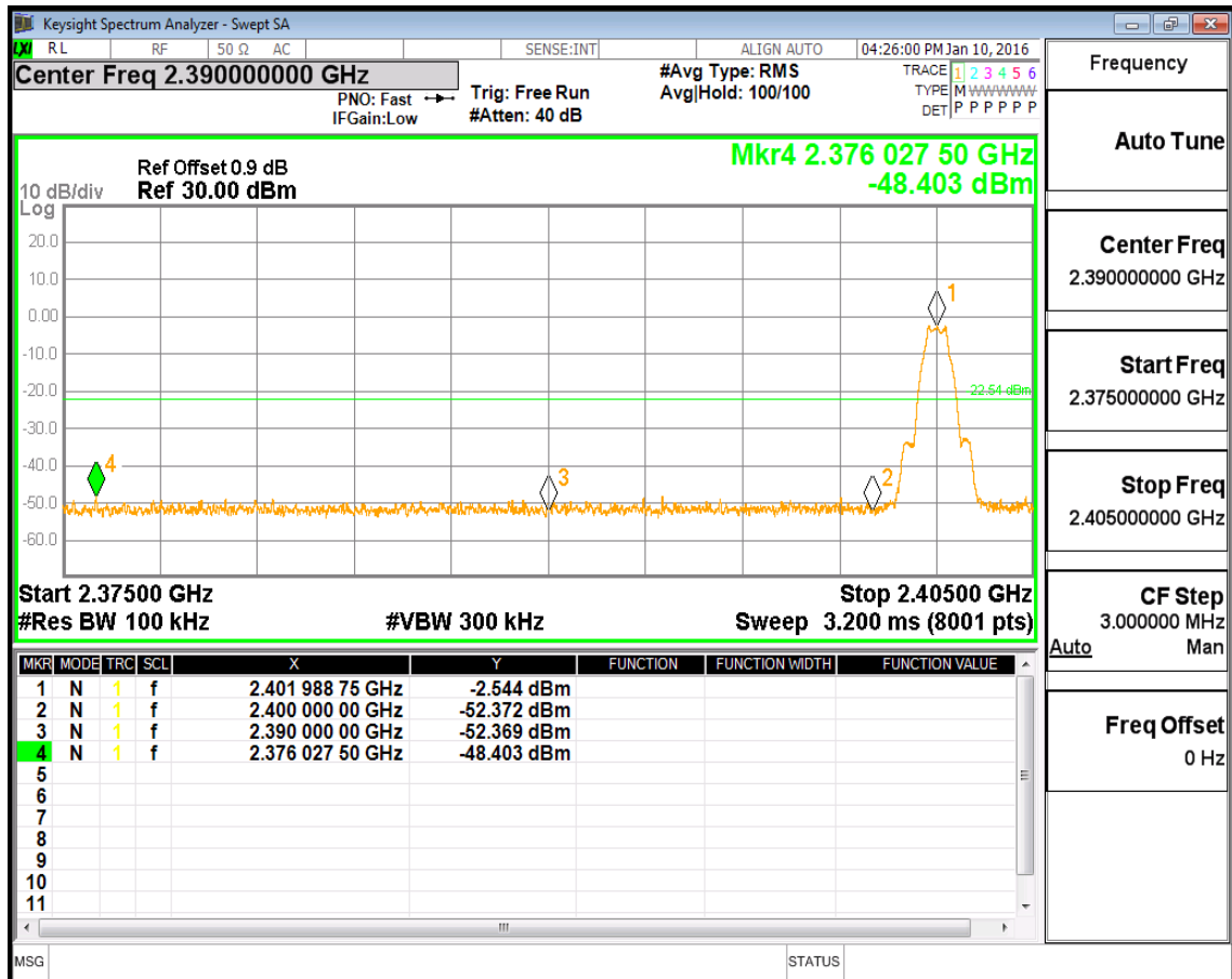
(Plot 4.5.1 D1: Left Band edge @ GFSK)
