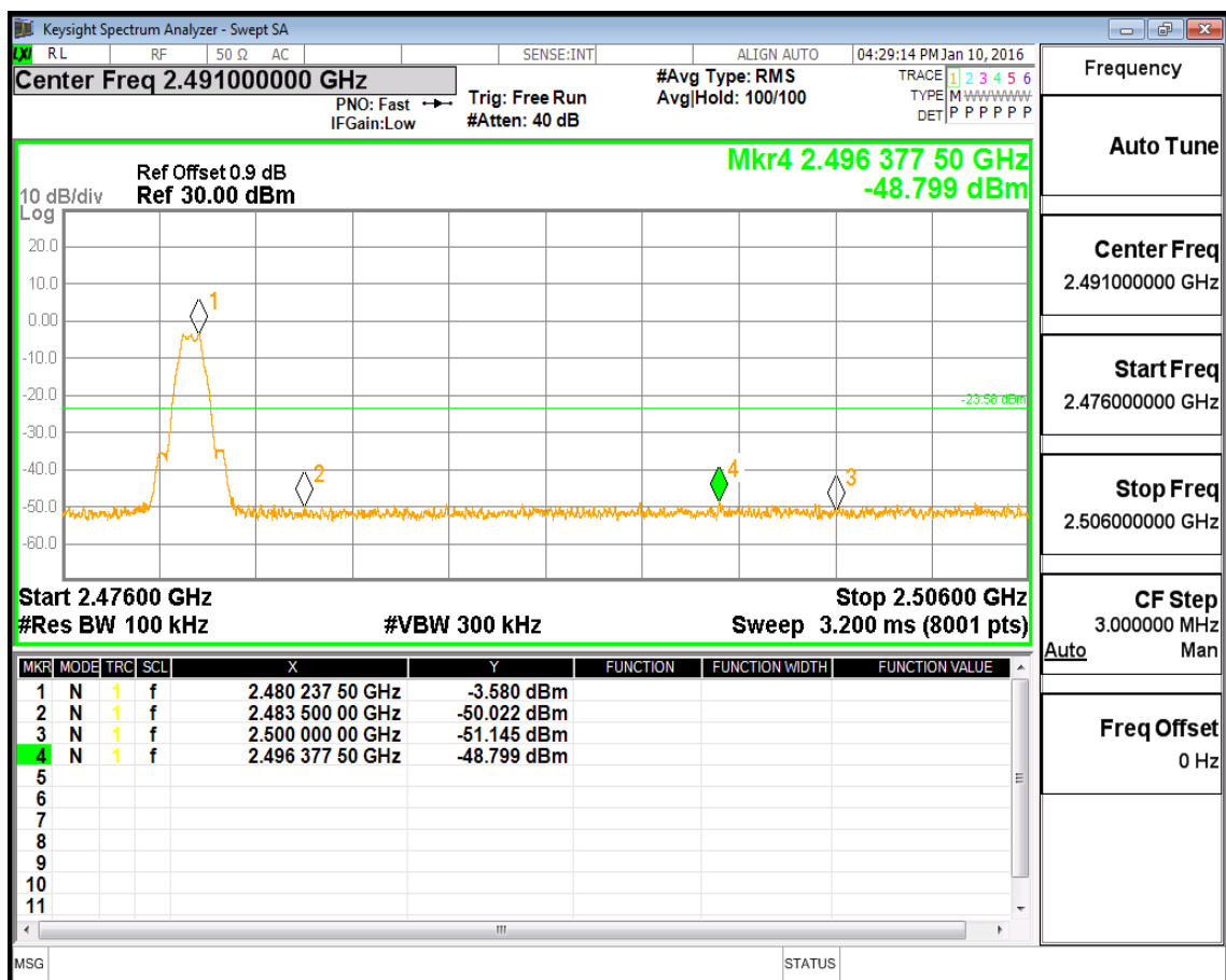
(Plot 4.5.1 D2: Right Band edge @ GFSK)
