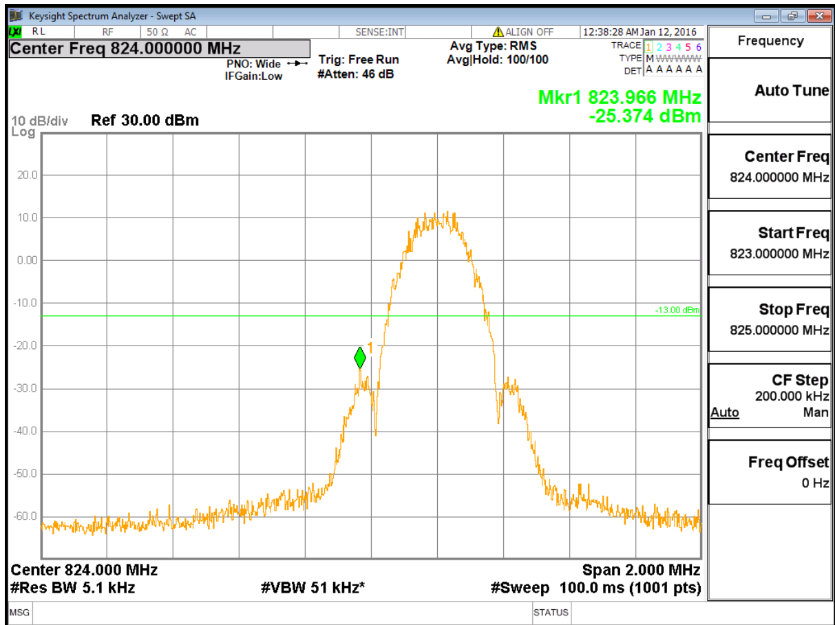
(Plot 4.4.2 A: Channel 128: 824.20MHz @ EGPRS850)
