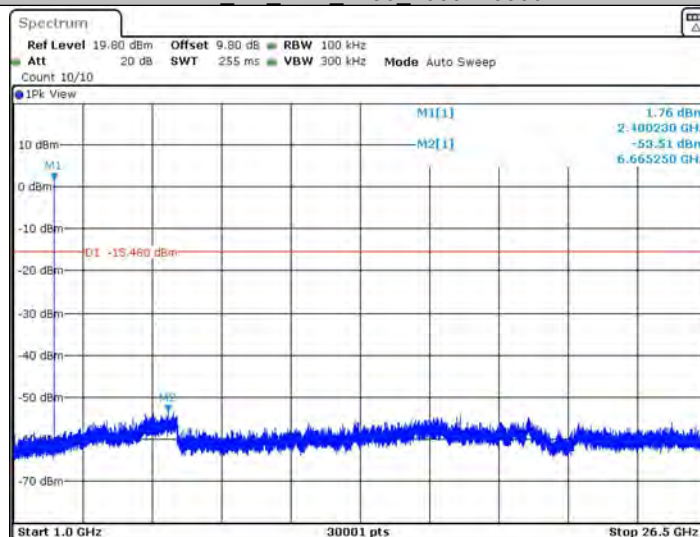
BLE_2M_Ant1_2480_1000~26500
