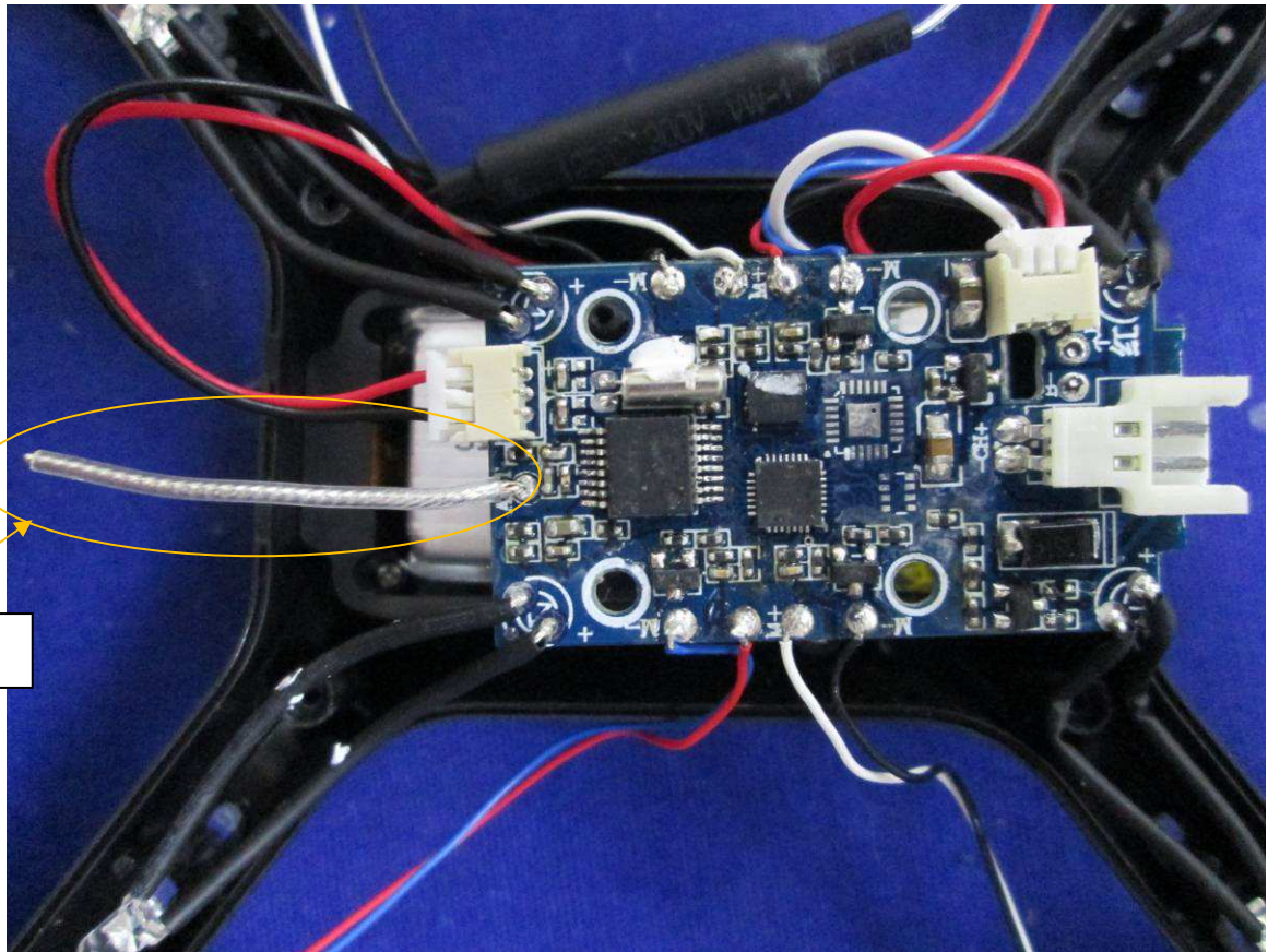
2.4G RX ANT
