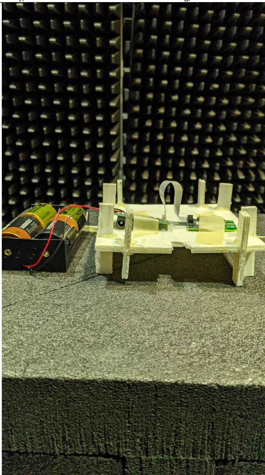
EUT Flat
