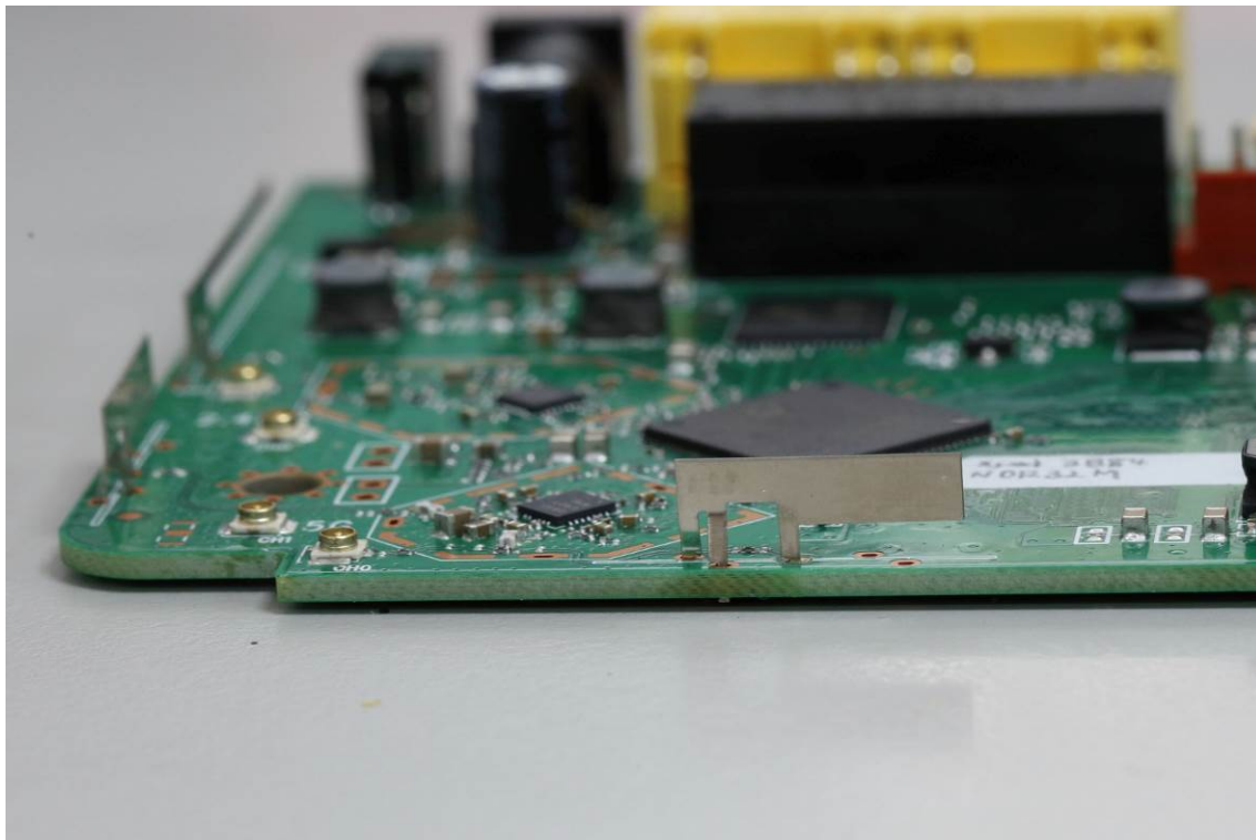
EUT 15 5G antenna 2
