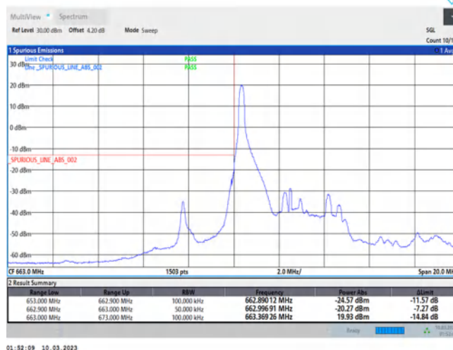
Band71-5MHz-QPSK-133147-25RB#0
